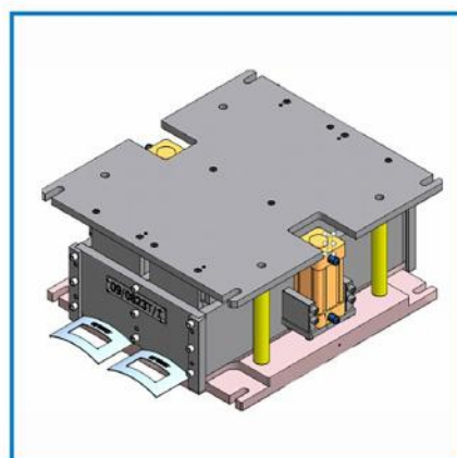
鼓式片预成型桶模 Preforming mold
